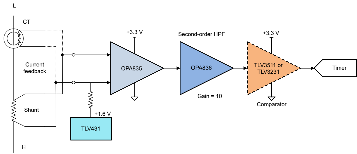
图 1. 典型应用：电弧故障检测
