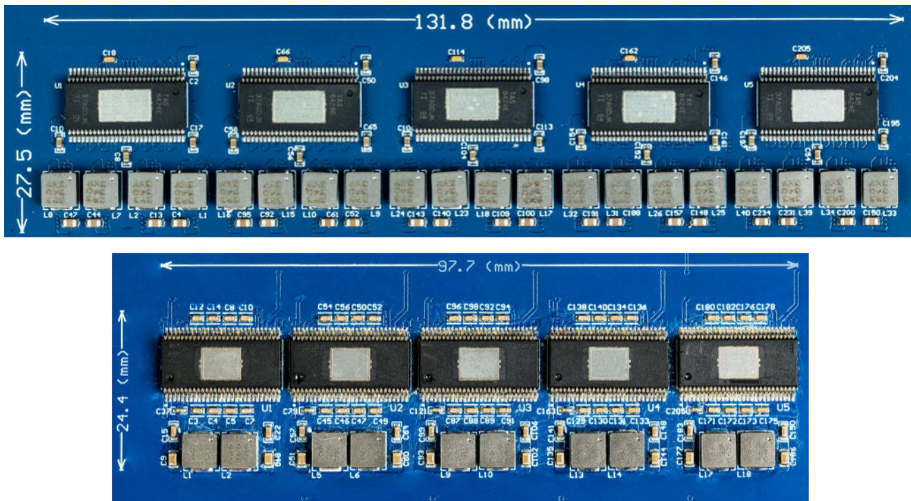
图 2. 一个采用 TI 的 TAS6424E-Q1 D 类放大器的 20 通道汽车音响系统设计 (上图)，与 TI 的 5 通道 TAS6754-Q1 D 类放大器 (下图) 之比较
