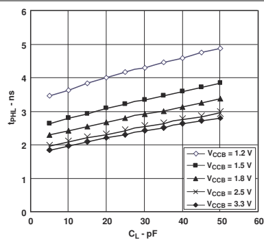
图 5-4. 典型 A 到 B 传播延迟, 从高电平到低电平
