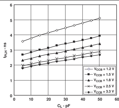
图 5-3. 典型 A 到 B 传播延迟, 从低电平到高电平
