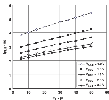
图 5-1. 典型 A 到 B 传播延迟, 从低电平到高电平
