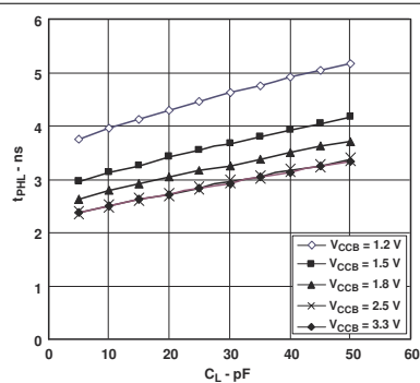
图 5-2. 典型 A 到 B 传播延迟, 从高电平到低电平
