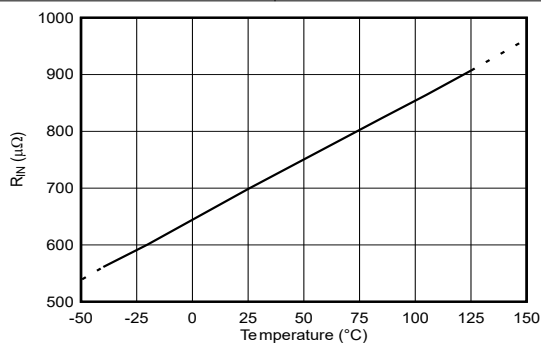
图 6-17. 输入导体电阻与温度间的关系
