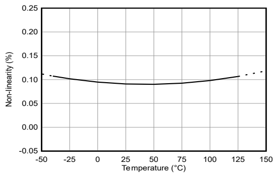
图 6-5. 非线性与温度间的关系
