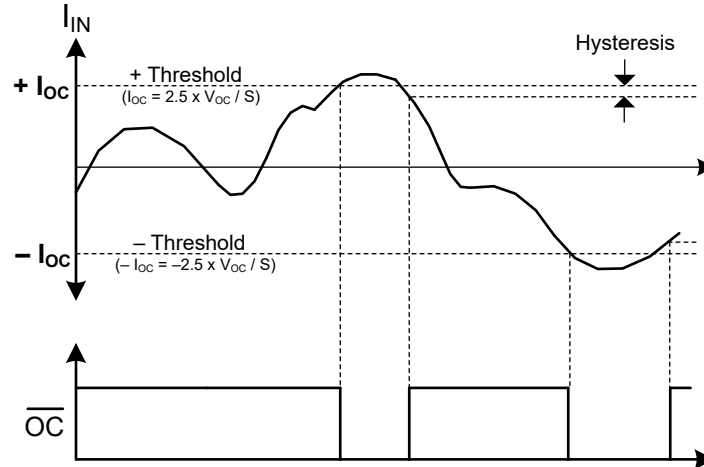
图 8-6. 过流输出响应
