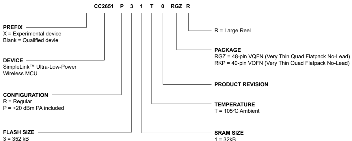
图 11-1. Device Nomenclature
