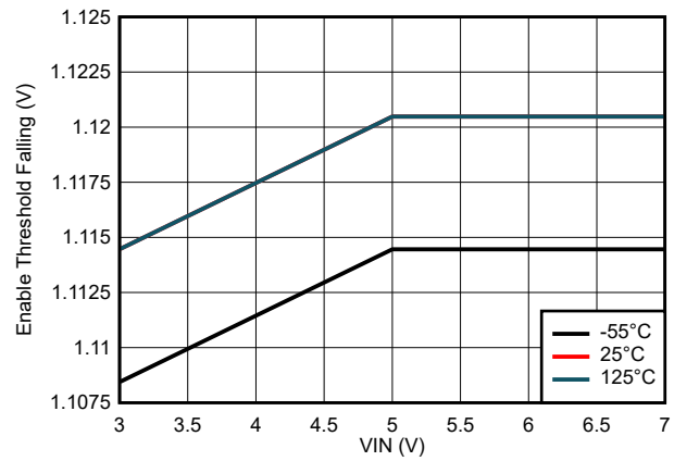
图 6-8. Enable Threshold Falling Variation
