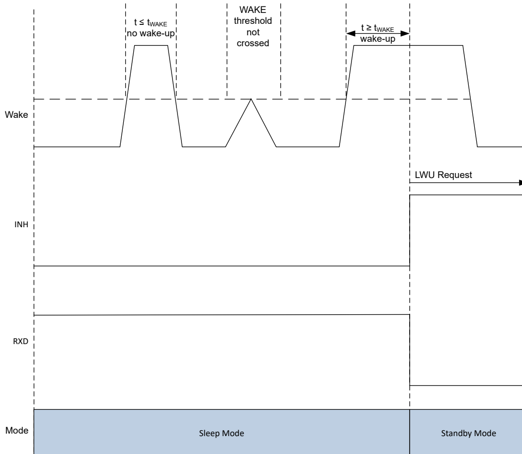
图 9-6. LWU Request Rising Edge
