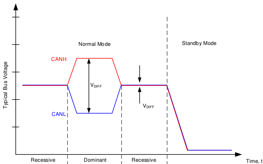
图 9-9. Bus States
