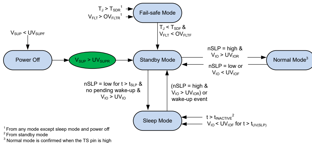
图 9-3. TCAN1162 State Machine
