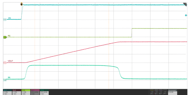
图 7-32. Input Hot-Plug
