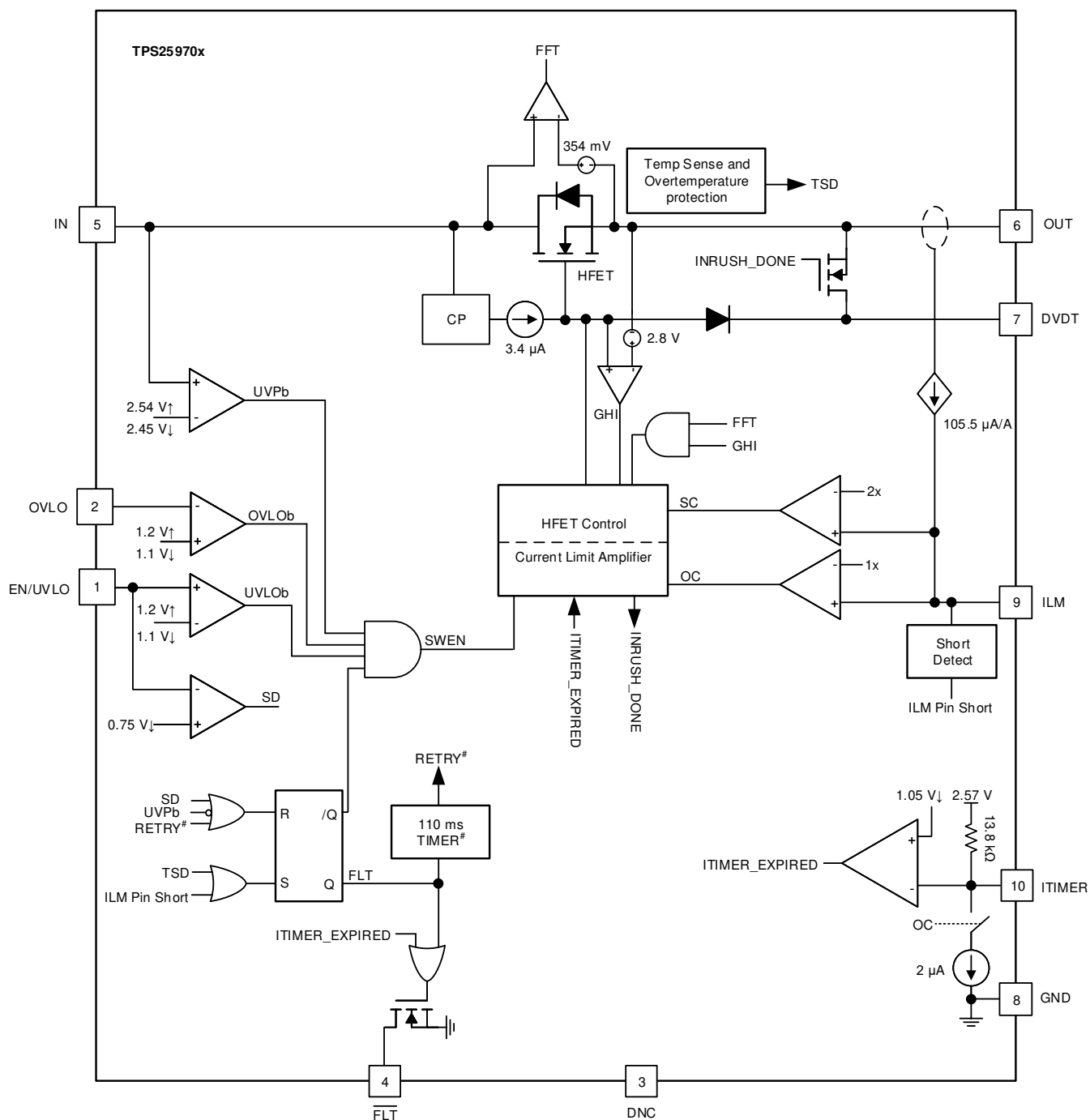
图 8-1. TPS25970x Block Diagram
