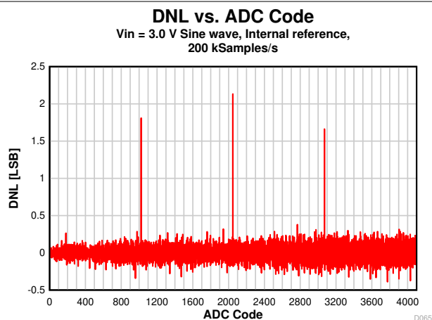
图 7-26. DNL vs. ADC Code
