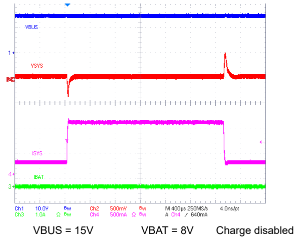
图 10-15. VSYS Load Transient Response
