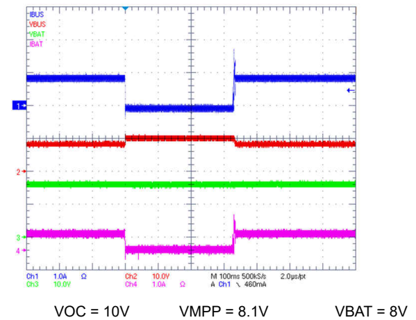
图 10-19. MPPT Operation Zoom
