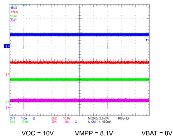
图 10-18. MPPT Operation
