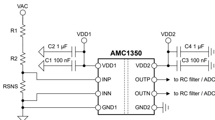
图 9-1. Decoupling of the AMC1350
