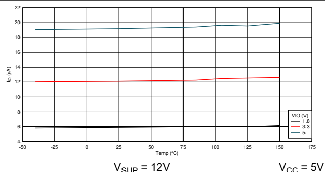
图 8-6. 正常模式： I_O 与温度间的关系 (显性)
