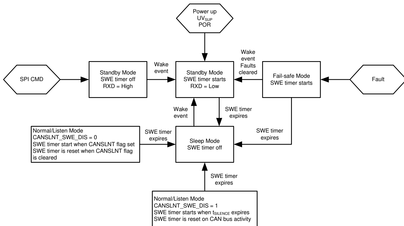
图 10-22. 睡眠唤醒错误 (SWE) 计时器
