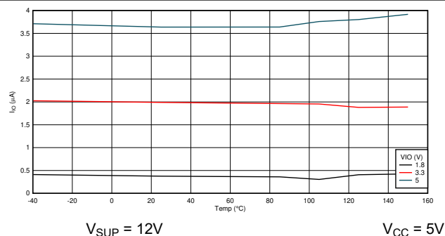
图 8-5. 正常模式： I_O 与温度间的关系 (隐性)
