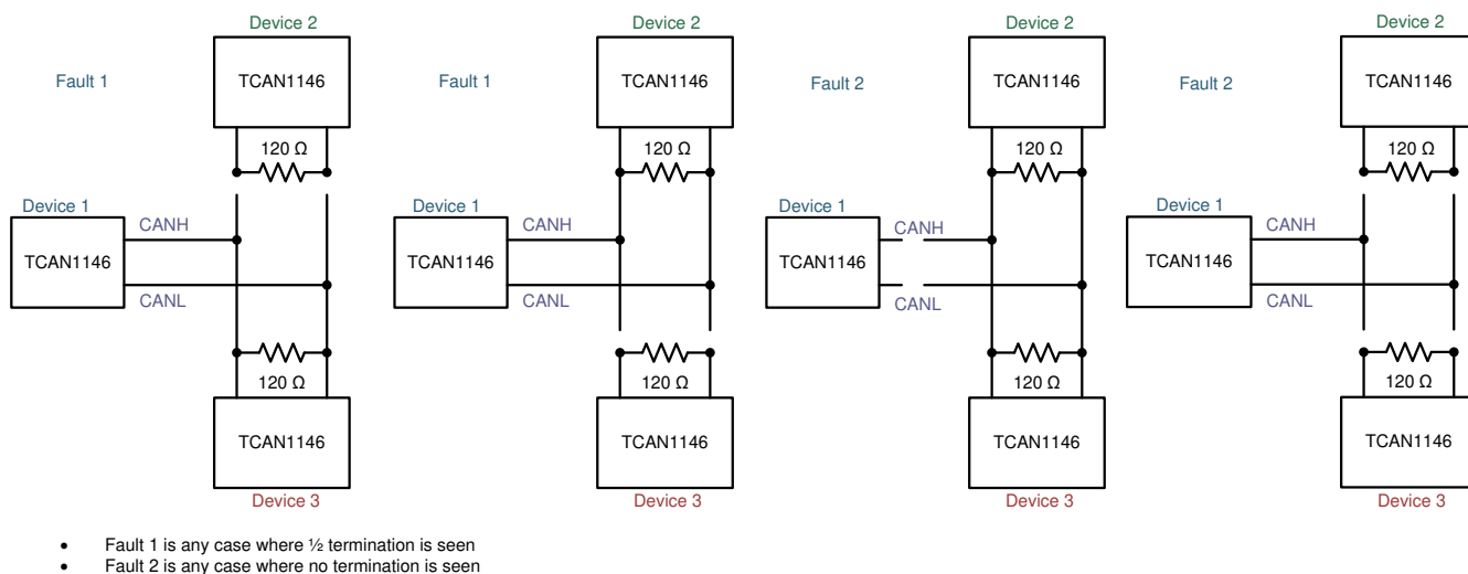
图 10-30. 开路故障 1 和 2 示例
