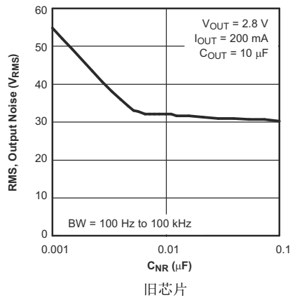
图 5-10. 均方根输出噪声与 C_{NR} 间的关系
