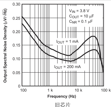
图 5-8. TPS793 输出频谱噪声密度与频率间的关系
