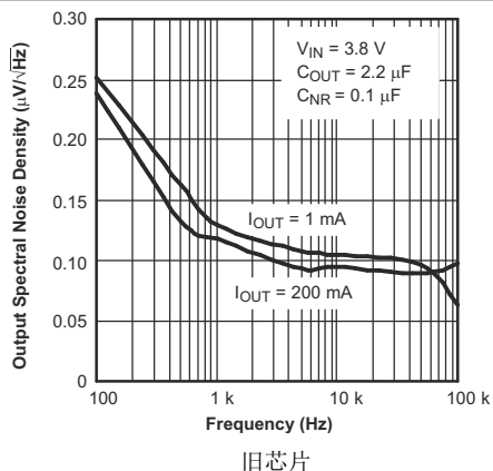
图 5-7. TPS793 输出频谱噪声密度与频率间的关系
