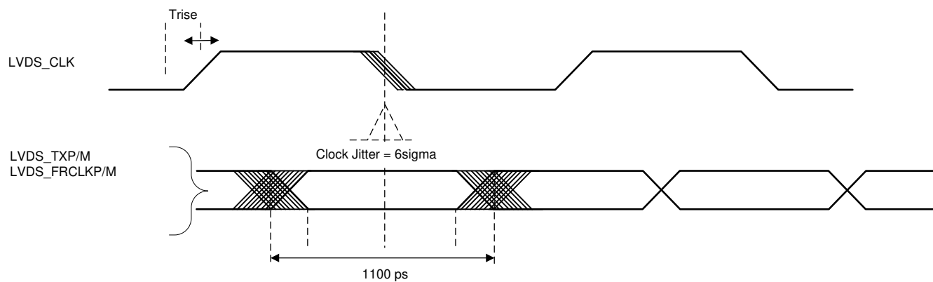
图 8-14. Timing Parameters
