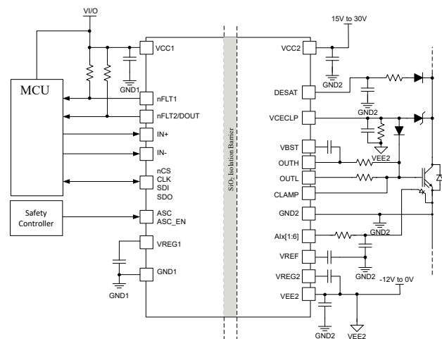
简化原理图
