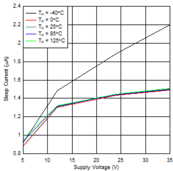
图 6-1. 睡眠电流与电源电压之间的关系
