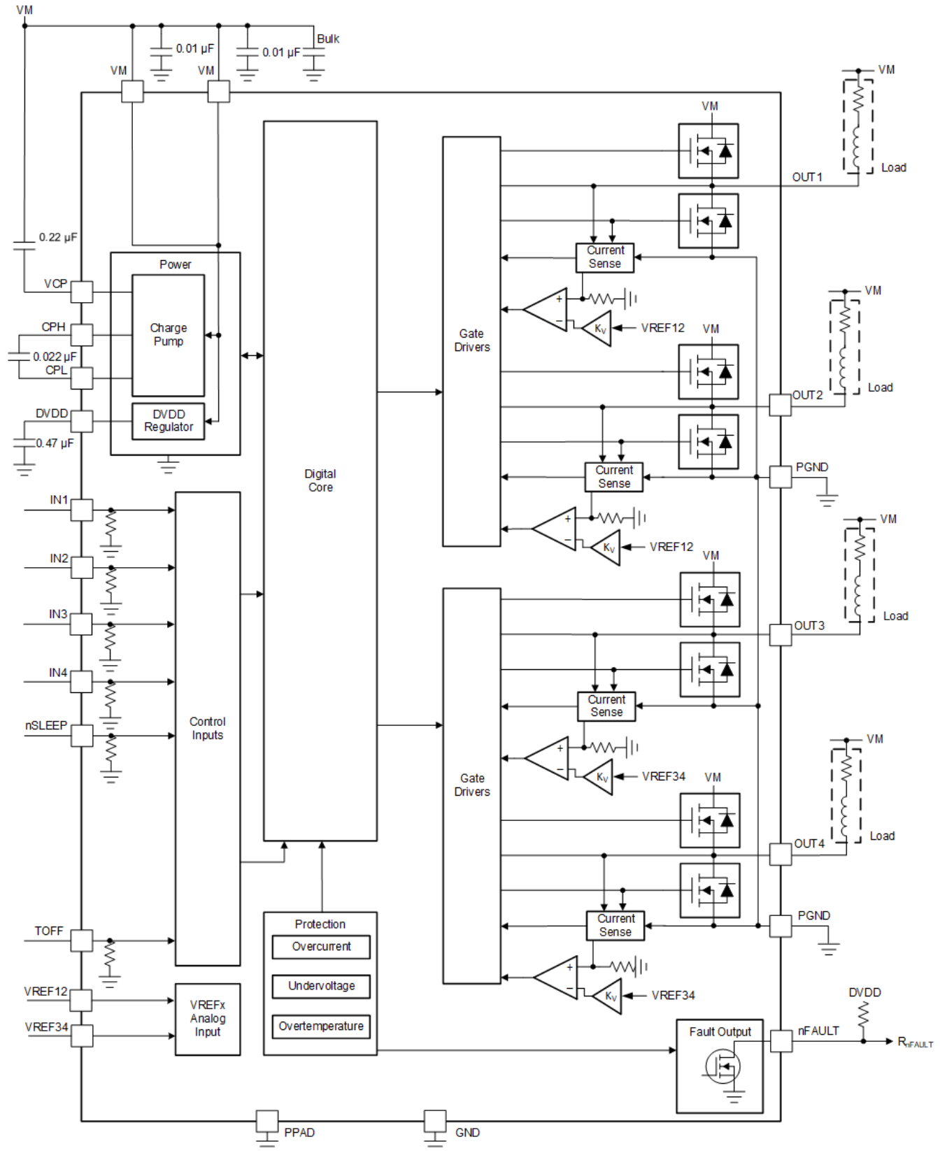
图 7-1. DRV8932 方框图
