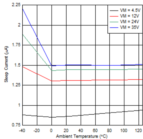
图 6-2. 睡眠电流与温度之间的关系
