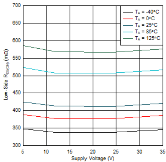
图 6-5. 低侧 R_{DS(ON)} 与电源电压之间的关系
