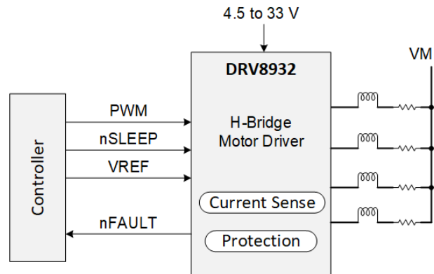
DRV8932 简化版原理图
