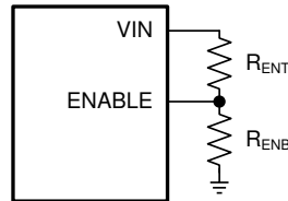
图 7-5. System UVLO
