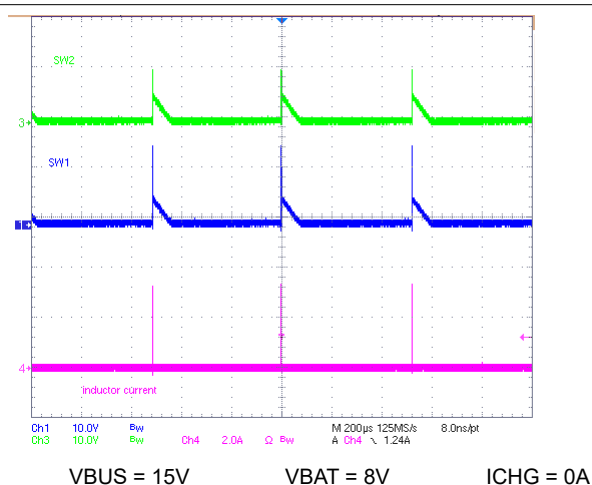
图 10-4. Buck Mode PFM without OOA
