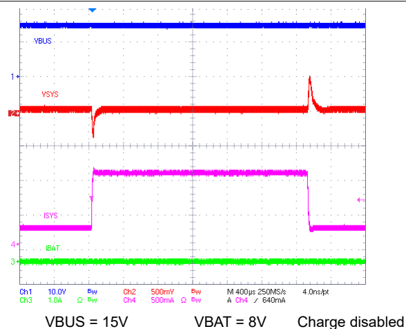
图 10-7. VSYS Load Transient Response
