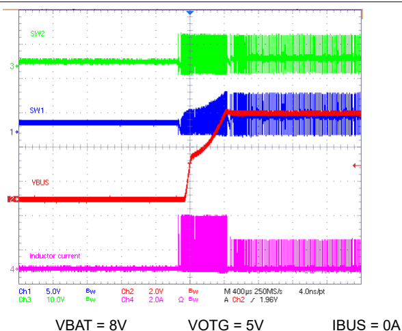
图 10-5. OTG Startup at No Load
