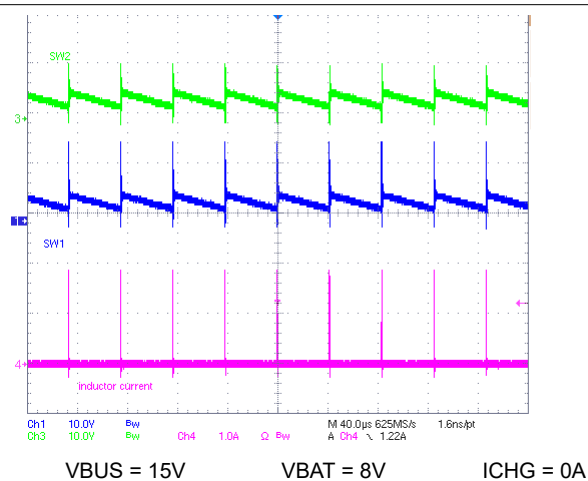
图 10-3. Buck Mode PFM with OOA
