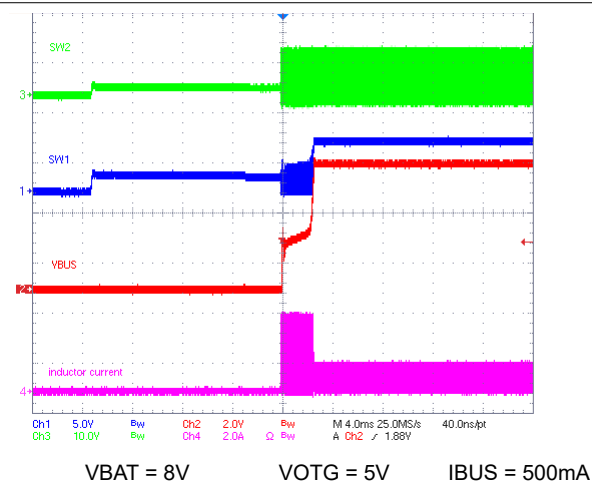
图 10-6. OTG Startup at 500-mA Load
