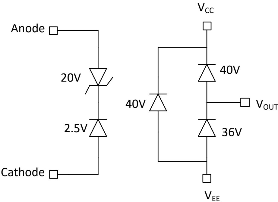
图 8-9. ESD Structure
