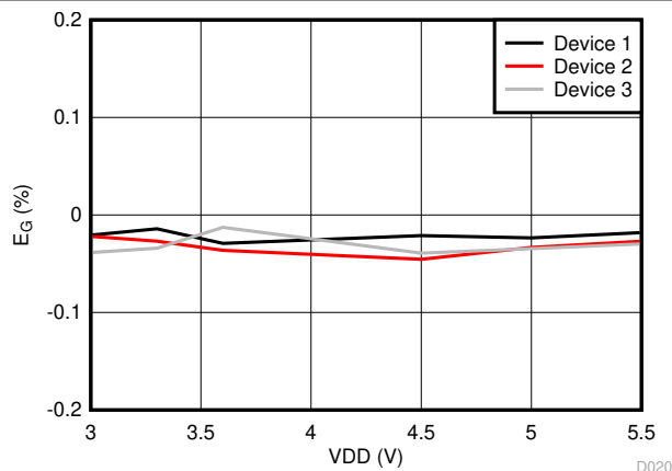
图 6-17. 增益误差与电源电压间的关系
