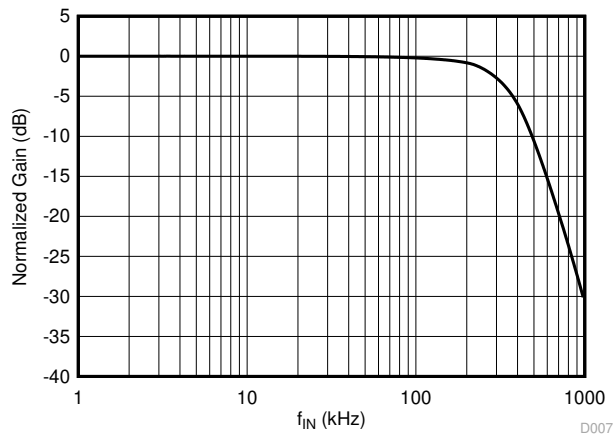
图 6-11. 归一化增益与输入频率间的关系
