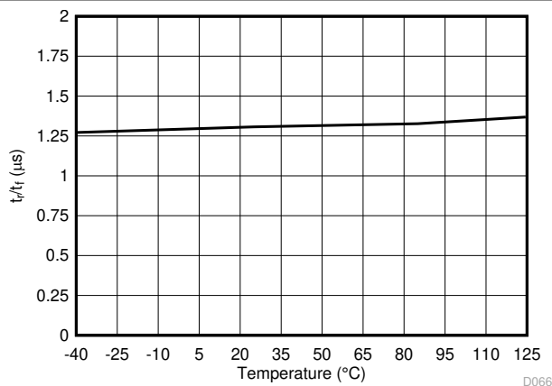
图 6-35. 输出上升和下降时间与温度间的关系
