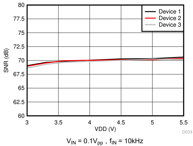
图 6-23. 信噪比与电源电压间的关系
