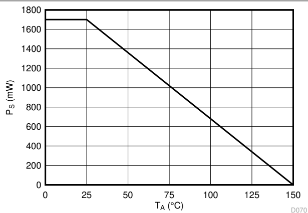
图 6-3. 安全限制功率的热降额曲线 (符合 VDE)
