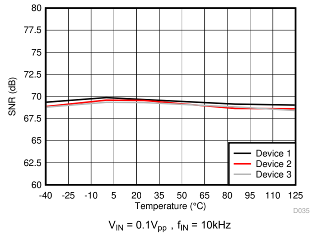
图 6-24. 信噪比与温度间的关系
