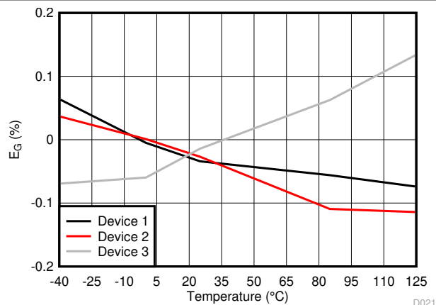
图 6-18. 增益误差与温度间的关系
