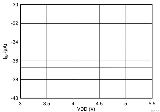
图 6-6. 输入偏置电流与电源电压间的关系
