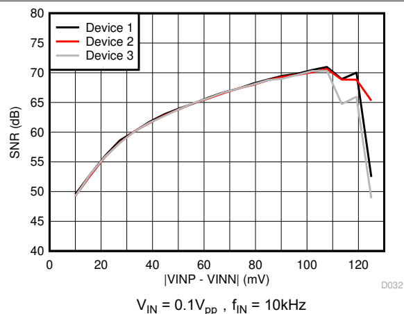
图 6-22. 信噪比与输入电压间的关系
