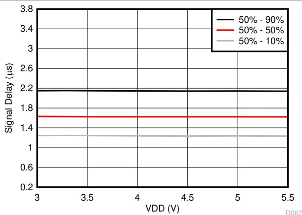
图 6-36. 从 V_{IN} 到 V_{OUT} 的信号延时与电源电压间的关系
