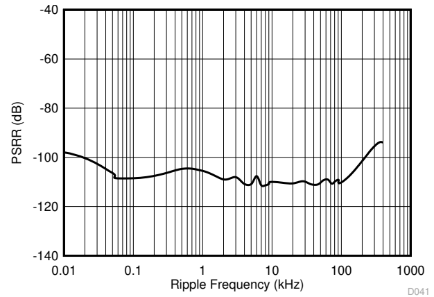
图 6-30. 电源抑制比与纹波频率间的关系
