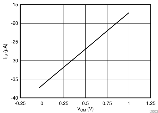
图 6-5. 输入偏置电流与共模输入电压间的关系
