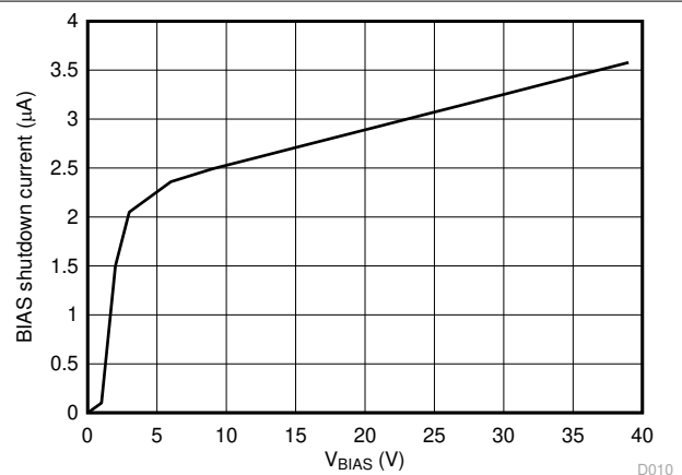
图 7-10. I_{\text{SHUTDOWN(BIAS)}} vs V_{\text{BIAS}}
