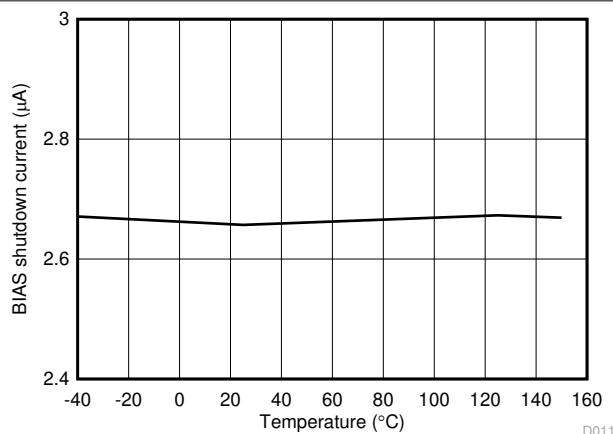
图 7-11. I_{\text{SHUTDOWN}} vs Temperature (BIAS = 12 V)
