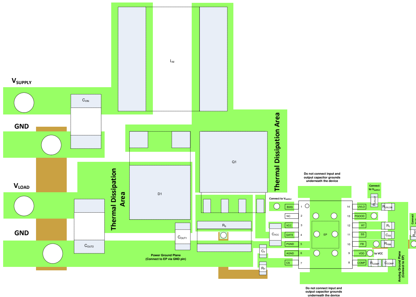
图 11-2. PCB Layout Example 2
