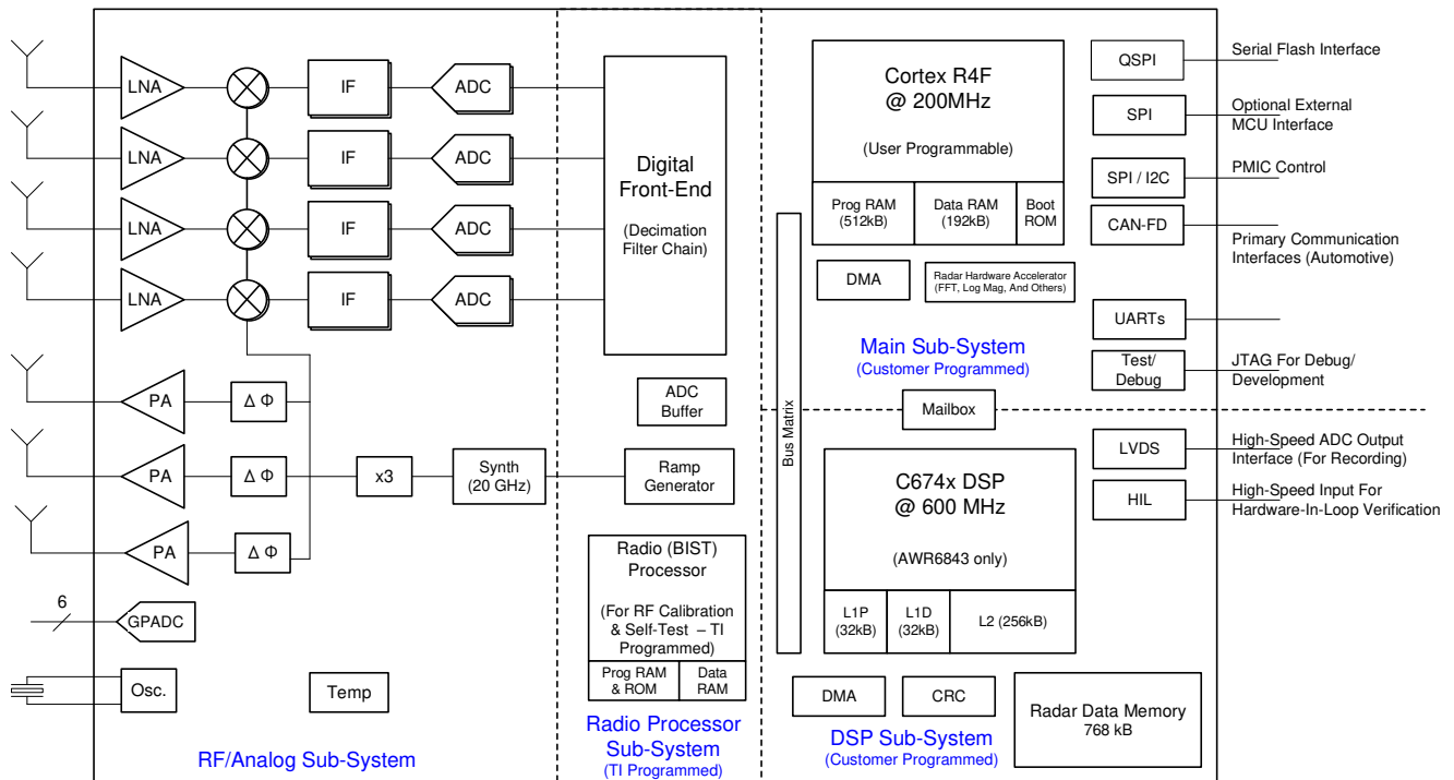
图 4-1. 功能方框图
