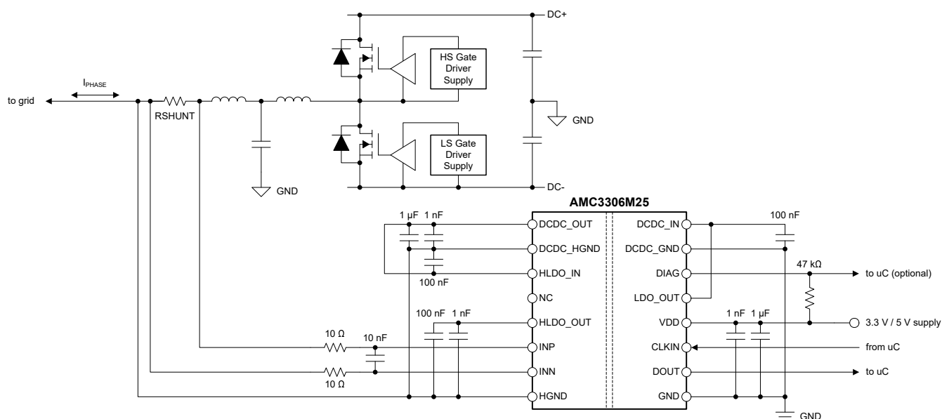
图 8-1. The AMC3306M25 在太阳能逆变器中的应用
