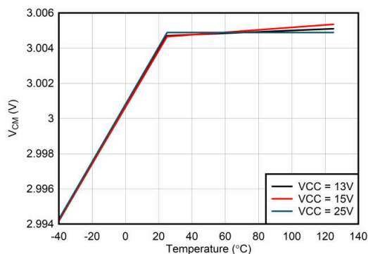
图 6-13. V_{\text{CM}} vs Temperature
