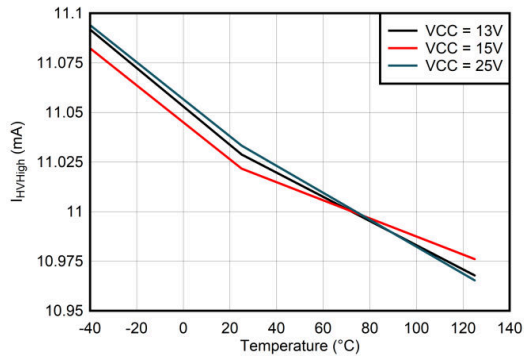
图 6-1. I_{HVHigh} vs Temperature
