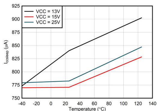
图 6-11. I_{\text{CCSleep}} vs Temperature
