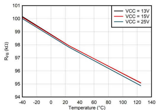
图 6-14. R_{\text{FB}} vs Temperature
