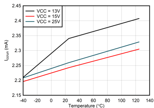
图 6-12. I_{\text{CCRun}} vs Temperature
