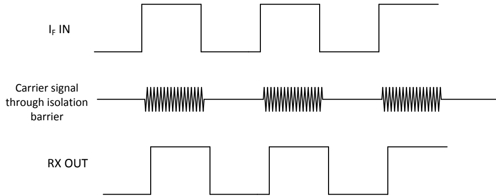
图 8-2. 基于关键控 (OOK) 的调制方案
