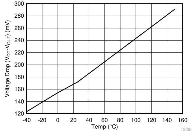
图 6-11. V_{OH} (20mA 负载) 与温度间的关系
