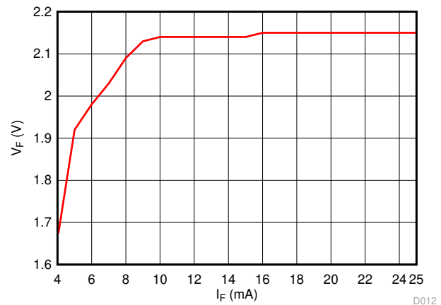
图 6-15. 正向电流与正向压降间的关系
