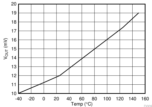
图 6-10. V_{OH} (无负载) 与温度间的关系
