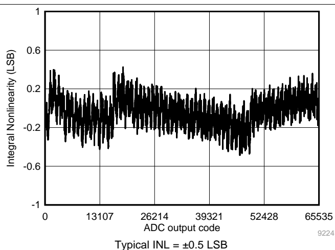
图 17. Typical INL
