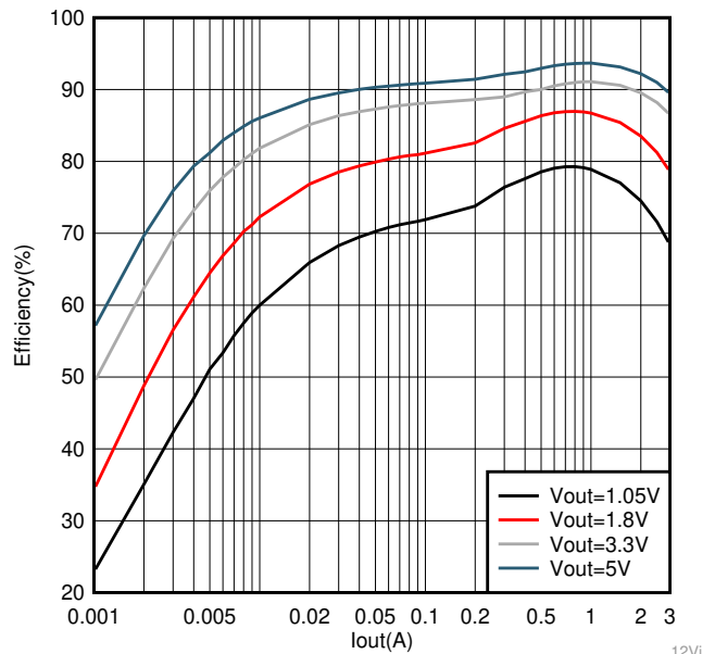
TPS563231 效率
