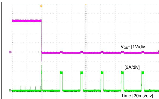
图 20. Short Protection
