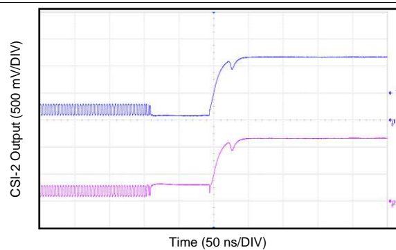
图 16. CSI-2 D0± End of Transmission
