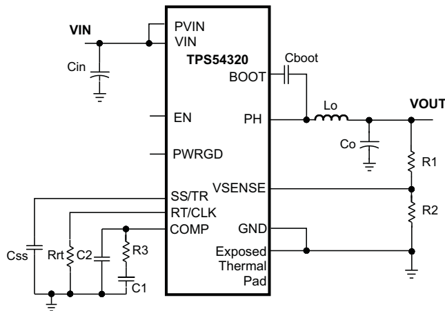
简化原理图
