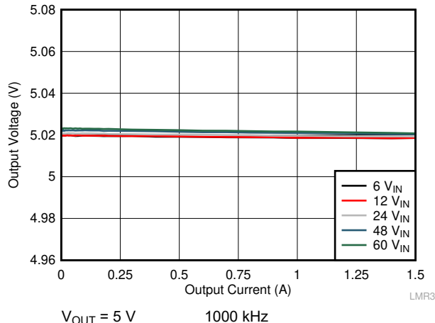
图 10-29. Load Regulation
