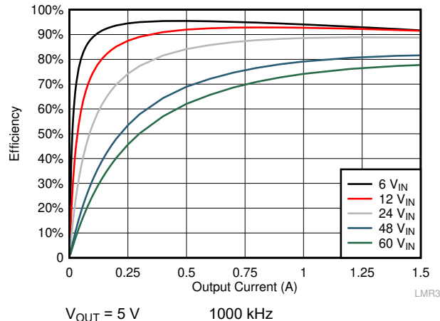
图 10-28. Efficiency
