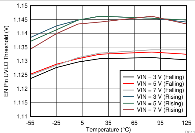
图 7. EN Pin UVLO Threshold vs Temperature
