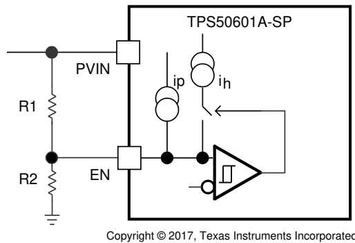
图 16. Adjustable PVIN UVLO
