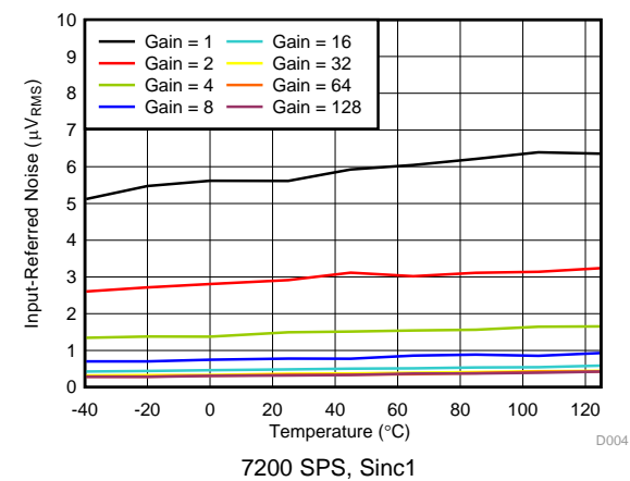
图 19. Noise vs Temperature
