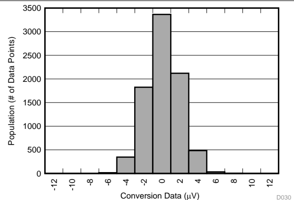
图 22. Conversion Data Histogram
