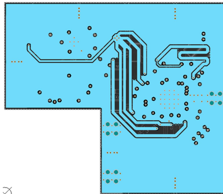
图 96. Mid Layer 1
