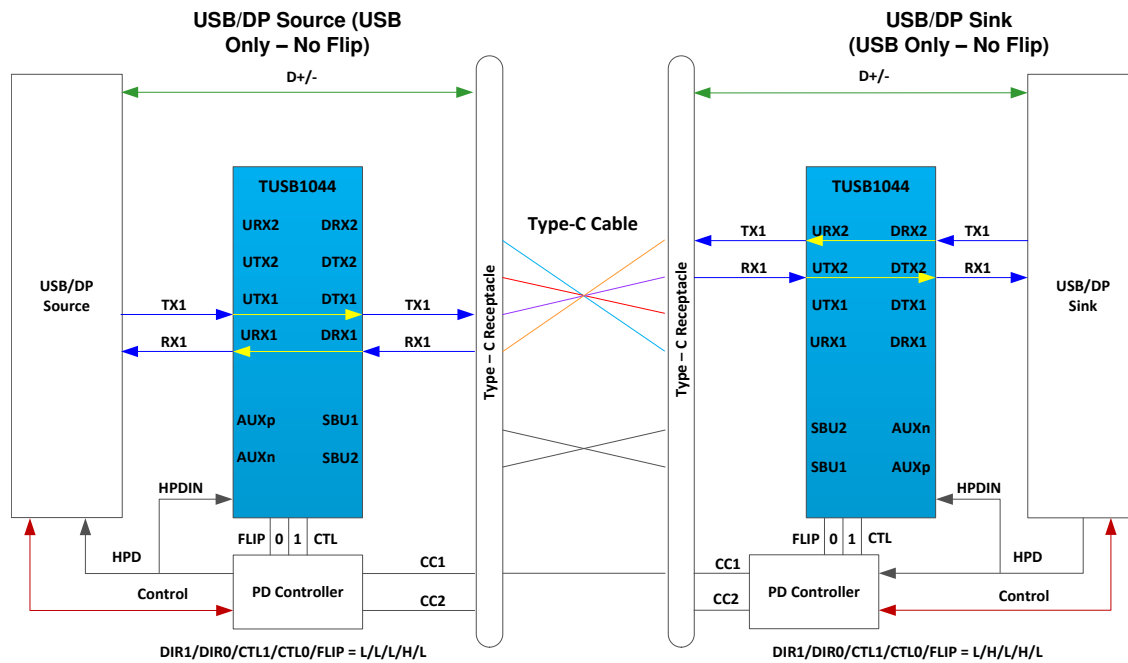
图 7-4. USB3.1 Only - No Flip
