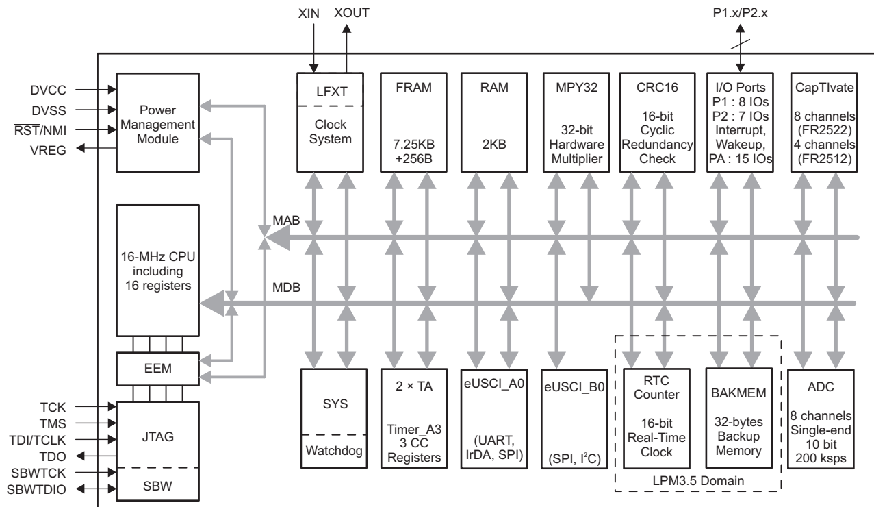
图 1-1. 功能框图
