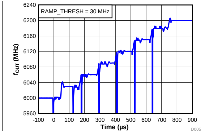
图 27. Automatic Ramping
