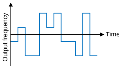
图 36. FSK Modulation
