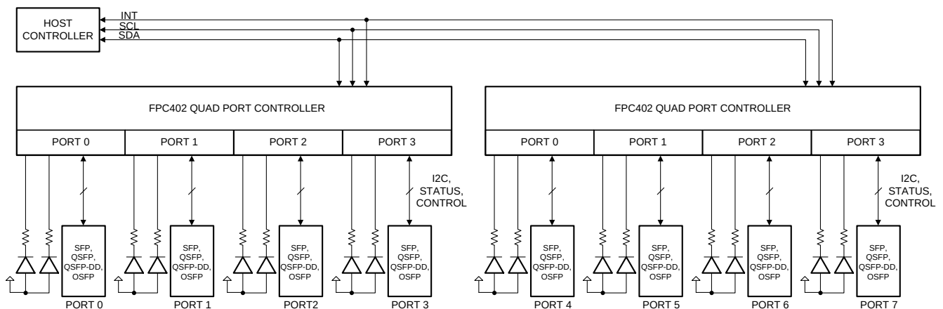
简化框图
