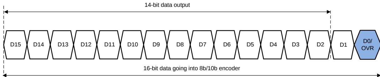
图 63. FOVR Timing Diagram
