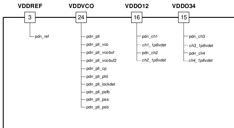
图 8-10. Power Management
