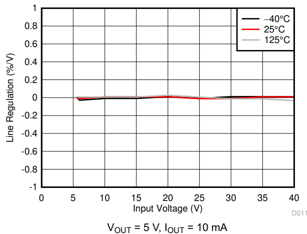
图 6-11. Line Regulation
