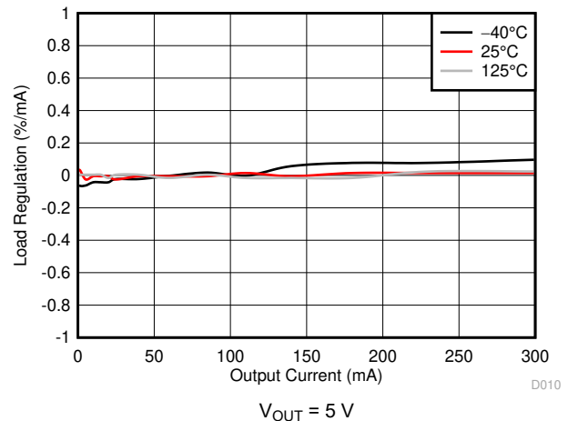
图 6-10. Load Regulation
