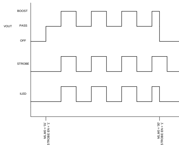
图 29. IR Mode with Boost
