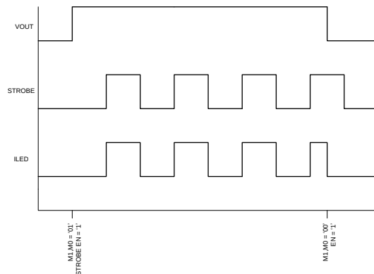
图 30. IR Mode Pass Only
