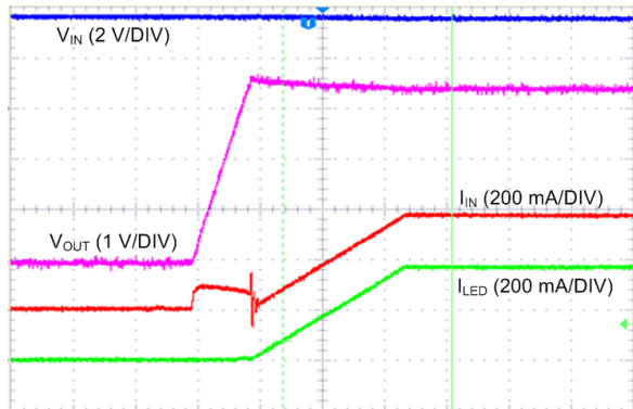
图 74. Pass Mode I 2 C Torch
