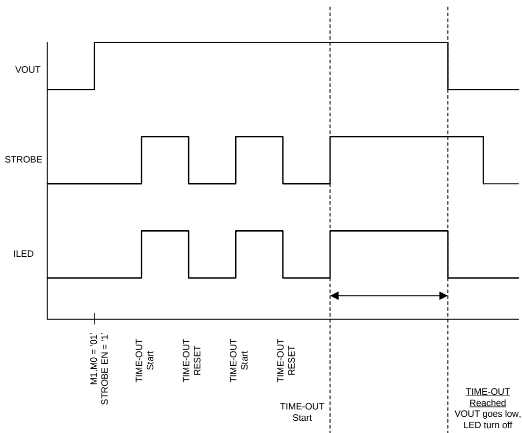
图 31. IR Mode Time-out
