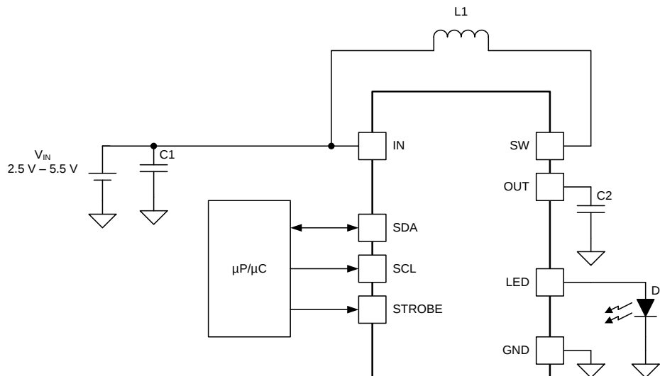
简化电路原理图
