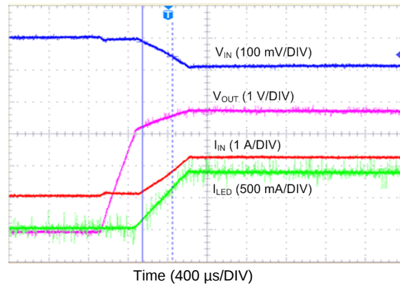
图 80. IVFM - Ramp and Hold
