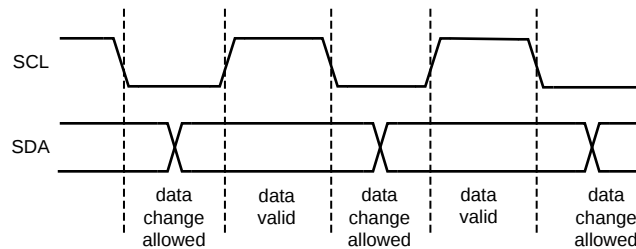
图 33. Data Validity Data
