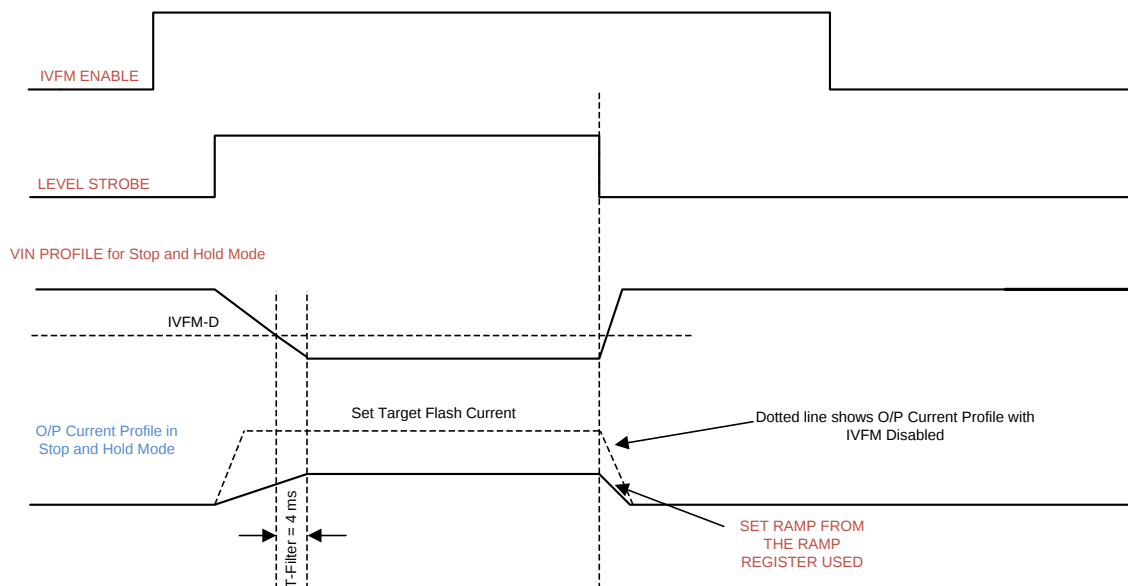
图 32. IVFM Mode
