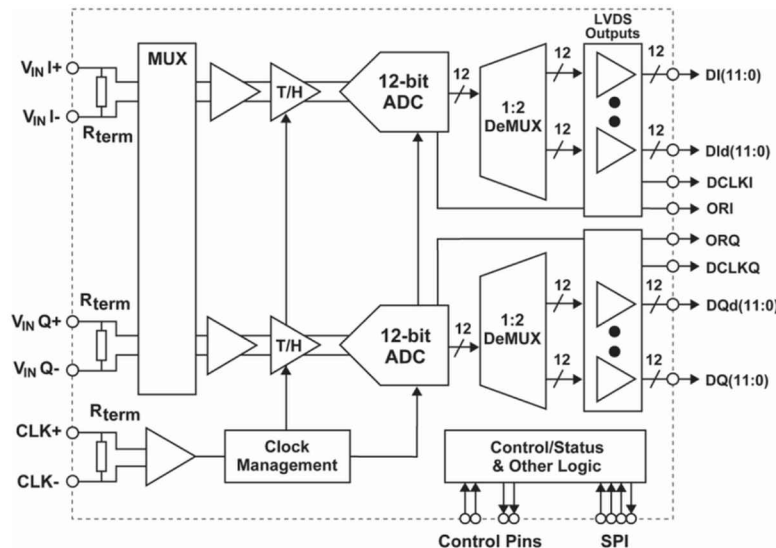
功能方框图
