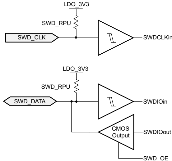
图 9-51. IOBUF_GPIOHSSWD
