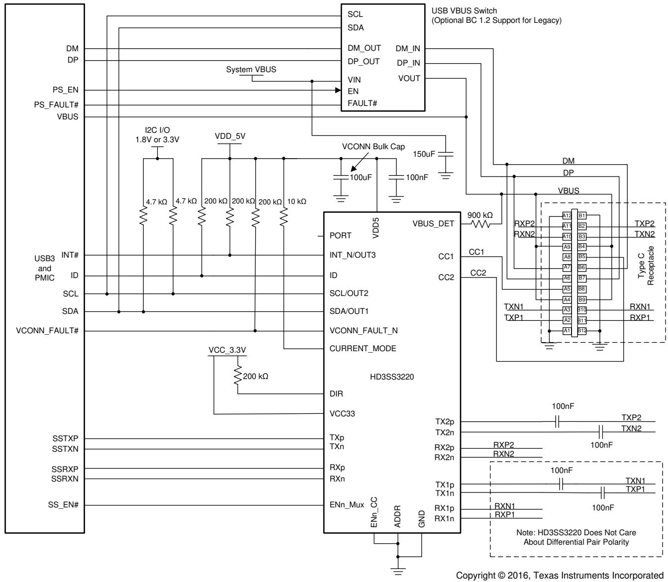
图 8-1. 使用 HD3SS3220 的 DRP 应用
