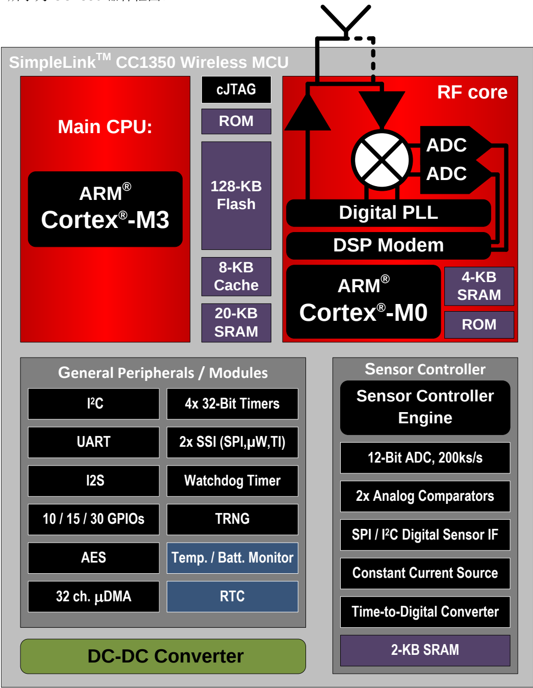
图 1-1. CC1350 框图
