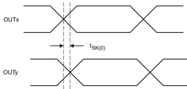
图 7-4. Output Inter-Pair Skew
