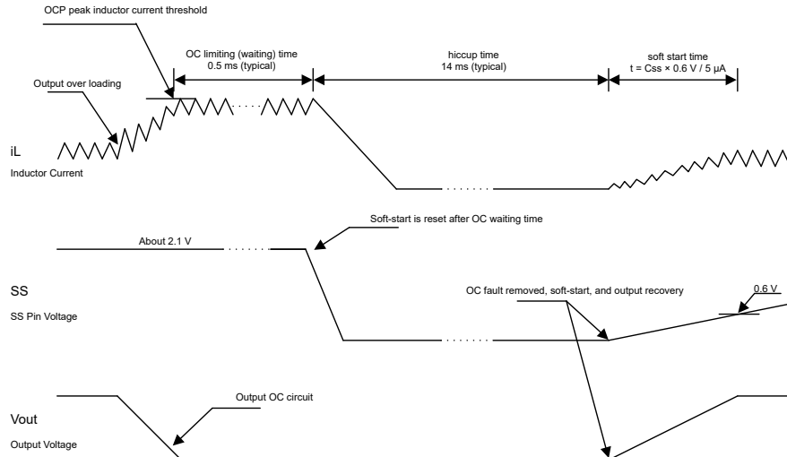
图 8-11. Overcurrent Protection
