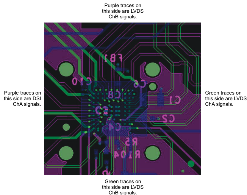
图 10-1. SN65DSI83 Layout Example
