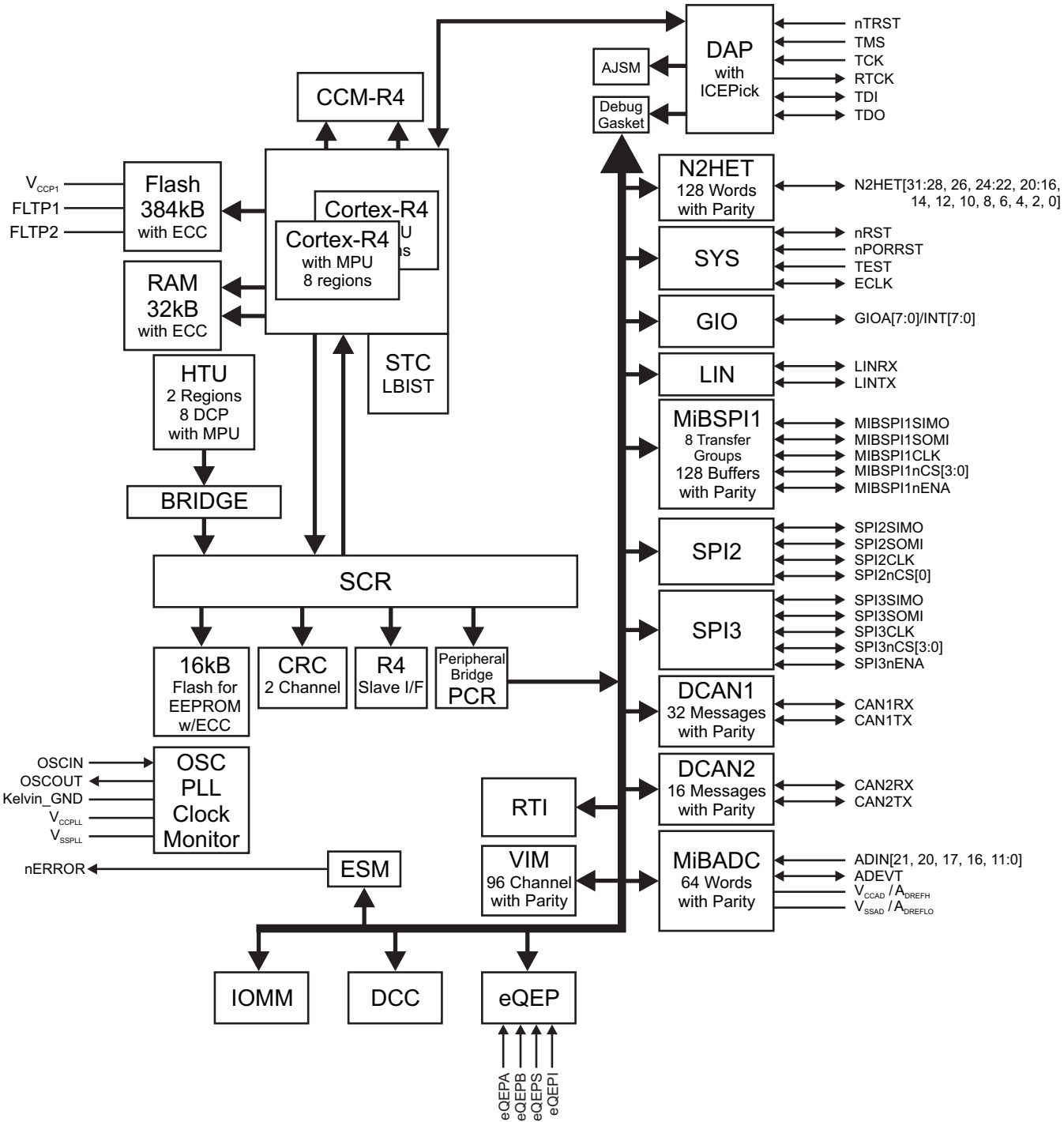
图 1-1. 功能方框图
