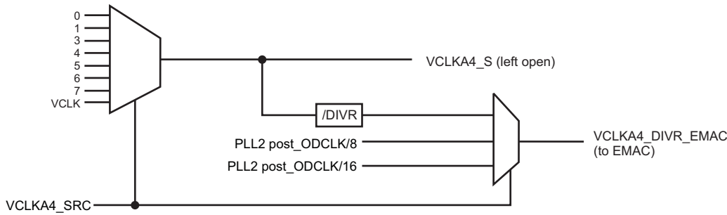
图 5-8. VCLKA4_DIVR 源选择选项
